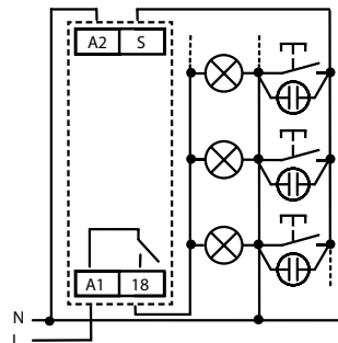
csatlakozás 4 vezetékkel
